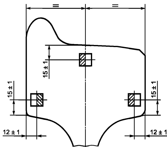
Рисунок 8 — Положение образцов для испытания на ударный изгиб в ободе колеса
